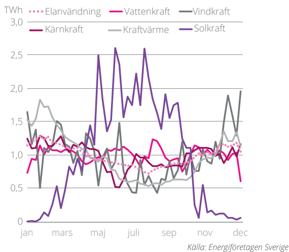
DIAGRAM 22 VECKOPROFILER FÖR ELANVÄNDNING OCH OLIKA KRAFTSLAG FÖR EL ÅR 2016
