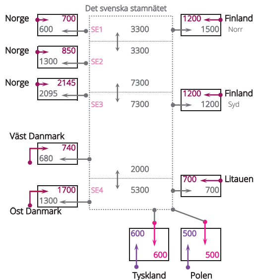
FIGUR 1 ÖVERFÖRINGSKAPACITET MELLAN SVERIGE OCH GRANNLÄNDERNA, MW
