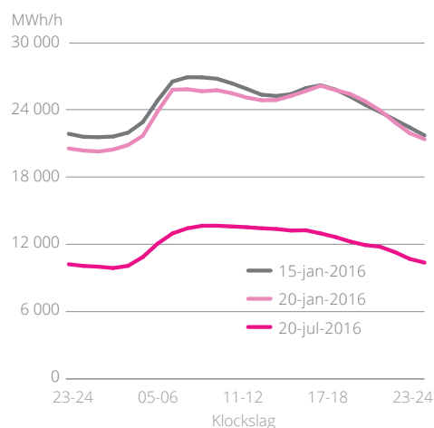
DIAGRAM 33 PROFIL ÖVER ELANVÄNDNING FÖR DYGN MED HÖGSTA ELANVÄNDNING UNDER EN TIMME, DEN 15 JAN 2016 RESPEKTIVE TYPDYGN VINTER OCH SOMMAR
