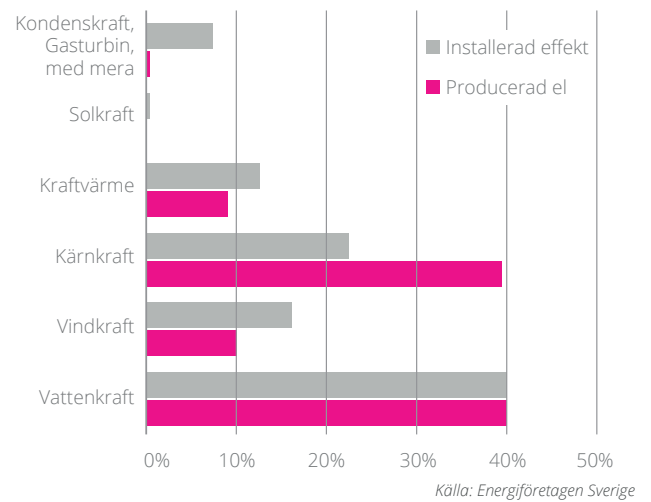
DIAGRAM 21 FÖRDELNING AV INSTALLERAD EFFEKT OCH PRODUCERAD EL FÖR OLIKA KRAFTSLAG ÅR 2016
