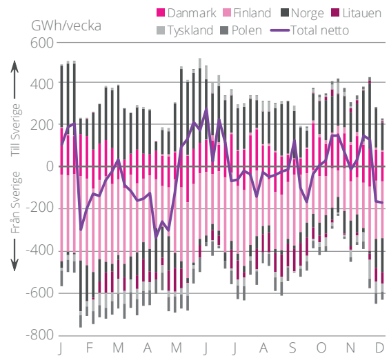
DIAGRAM 34 NETTOFLÖDE AV EL PER GRANNLAND TILL OCH FRÅN SVERIGE ÅR 2016, GWh/VECKA
