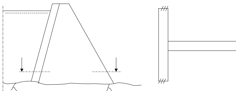
Lamelldamm - Sektion
