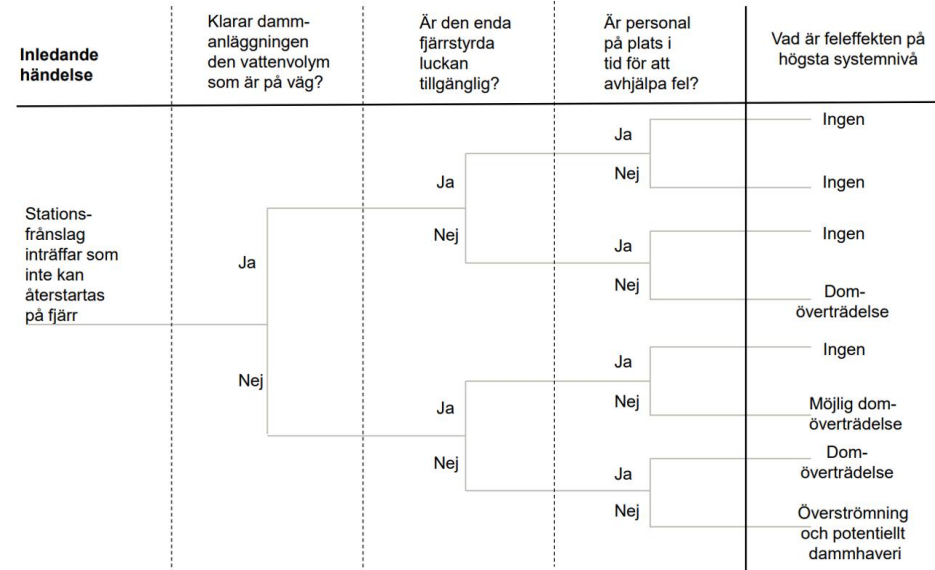
Figur 12. Exempel på händelseträdsdiagram för stationsfrånslag som inledande händelse
