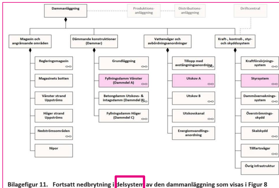
Bilagefigur 11. Fortsatt nedbrytning i delsystem av den dammanläggning som visas i Figur 8
