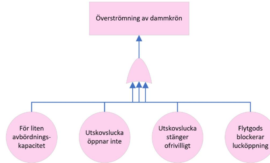
Figur 11. Exempel på ett felträdsdiagram
