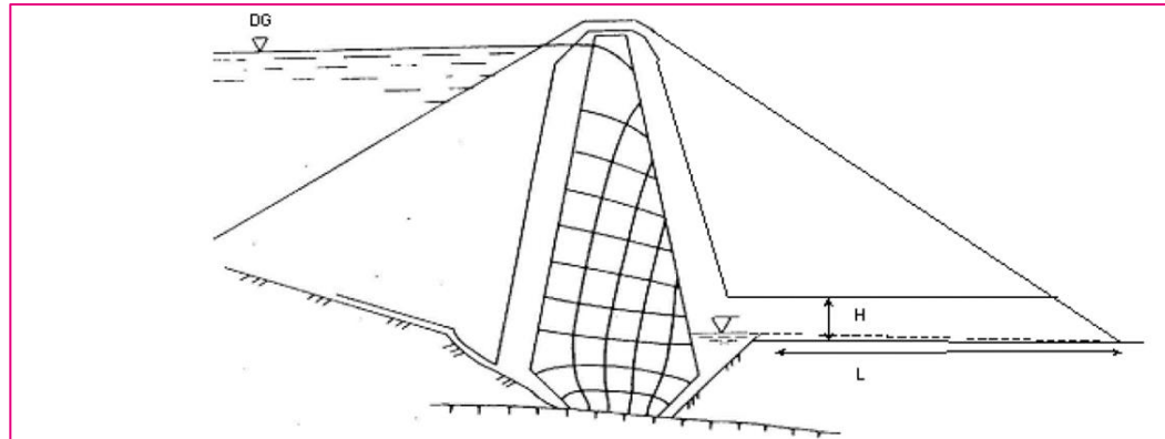
Bilagefigur 9. Modell över tryckfall i dammkroppen vid normal vattenströmning
